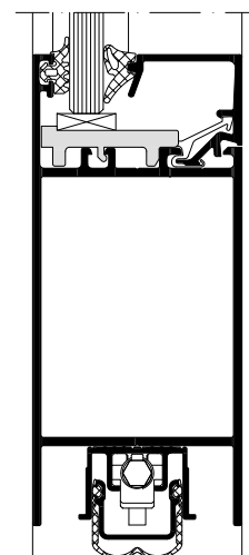
Schüco Дверь ADS 50.NI, масштаб 1:2 Schüco Door ADS 50.NI, scale 1:2
